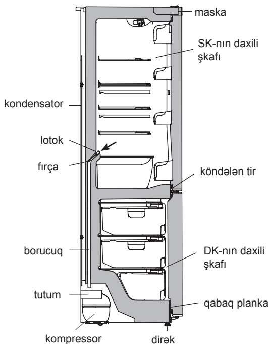
Şəkil 5 — Ərimiş suyun DK-dan axılması sxemi
